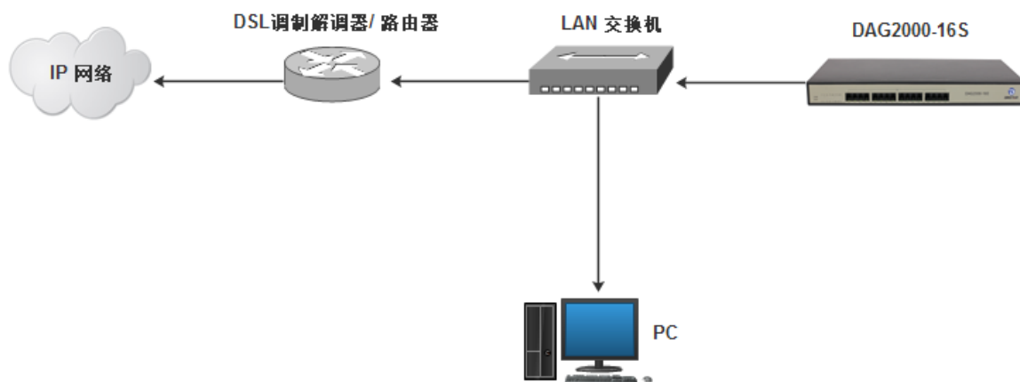
4.1-1 典型网络拓扑连接图
