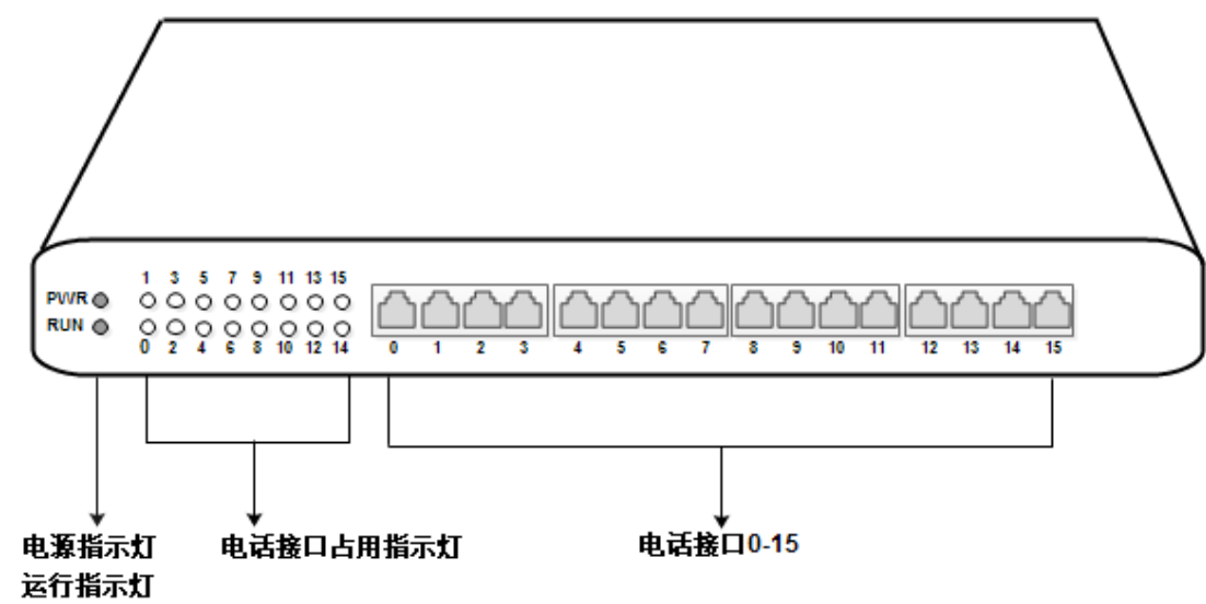
DAG2000-16S 指示灯说明
