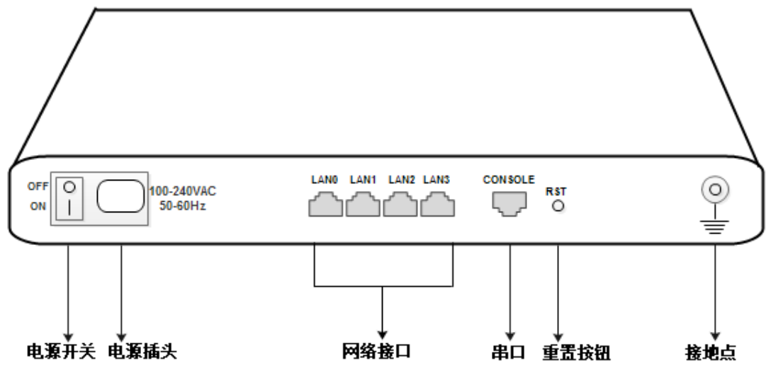
DAG2000-16S 接口和按钮说明
